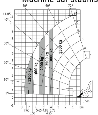
Machine sur stabilisateurs avec fourches
