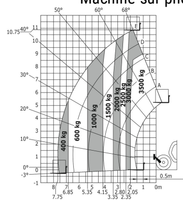
Machine sur pneus avec fourches
