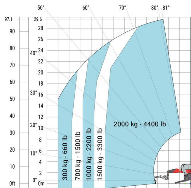
Machine sur stabilisateurs abaissés avec potence 2000 kg (Métrique)
