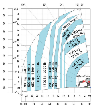
Machine sur stabilisateurs abaissés avec fourches
