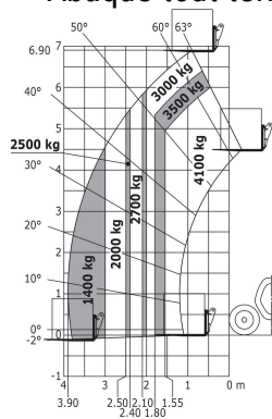
Abaque tout terrain (EN 1459 B)
