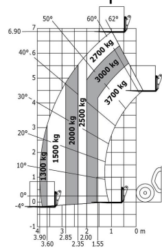
Abaque tout terrain (EN 1459 B)
