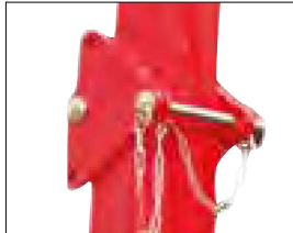
Châssis repliable pour la manipulation sous des toits.
